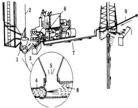
1-下灰漏斗；2-供灰罐；3-水的喷射；4-快速下灰；5-固井泵吸灰浆； 6-向套管内注入泥浆；7-水和水泥混合成水泥浆情况；8-钻井液循环管线
