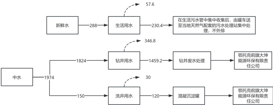
图 1 项目给排水平衡图 (单位: m 3 )
